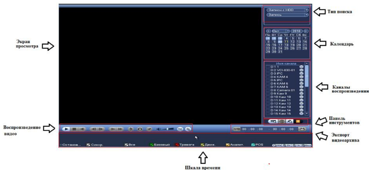
Рисунок 8.2 Интерфейс настройки пункта меню «Архив»
