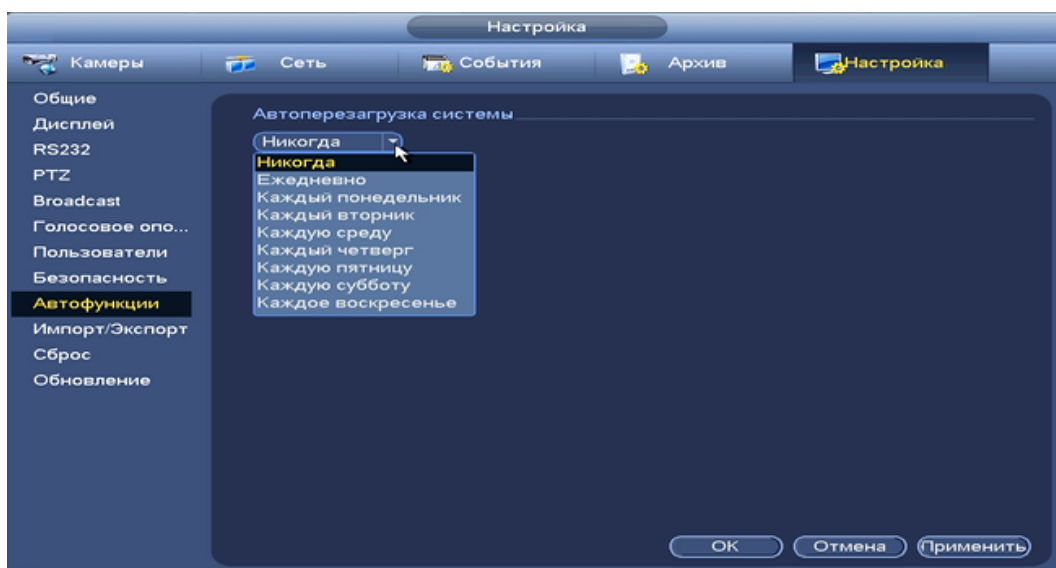
Рисунок 8.198 Интерфейс настройки автофункции.
