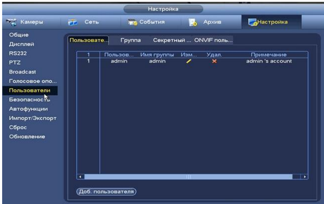
Рисунок 8.190 Интерфейс просмотра учетной записи.
