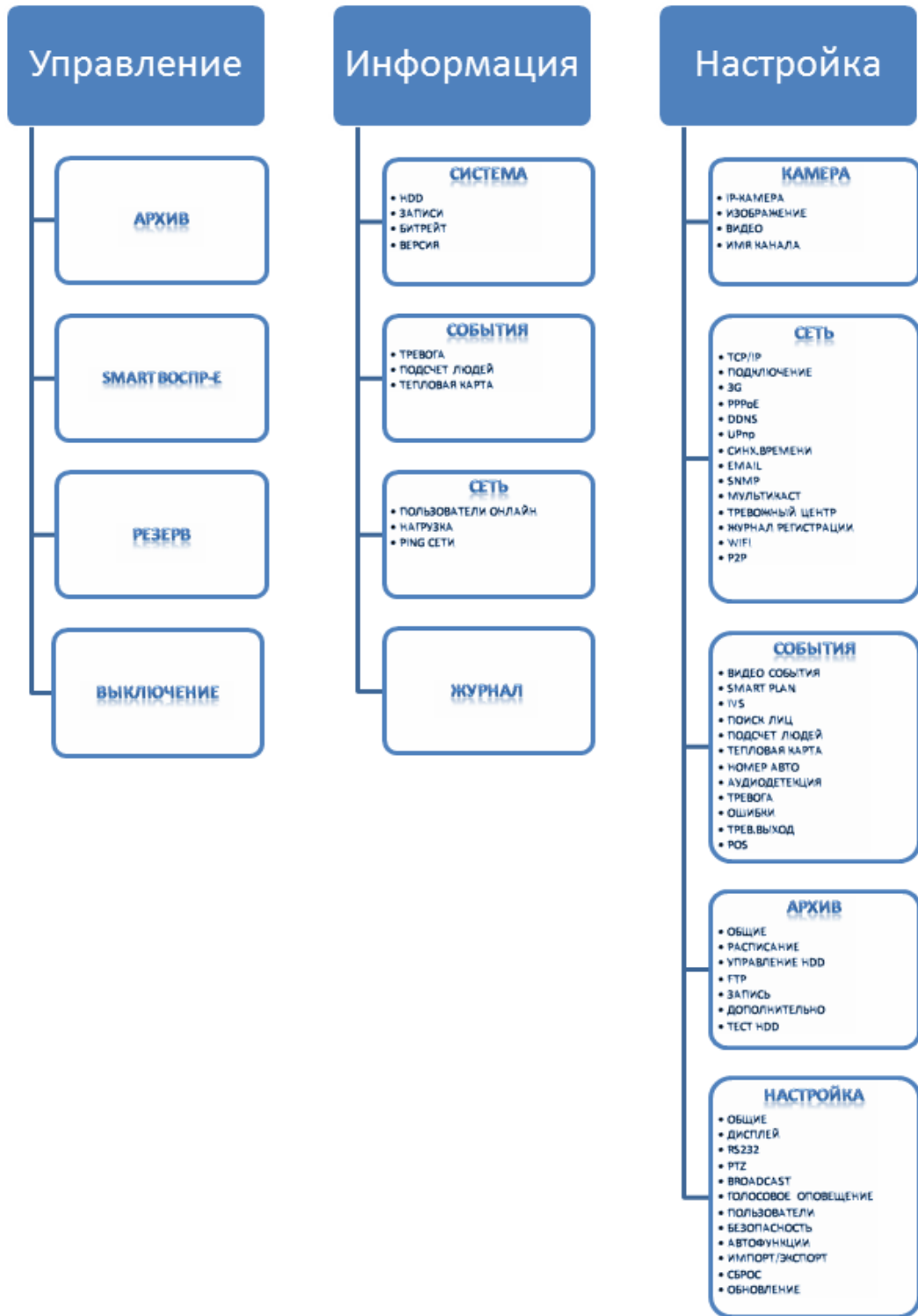
Рисунок 8.1 Схема главного меню.
