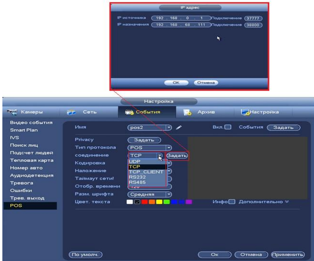
Рисунок 8.158 Ввод IP и протокола соединения.
