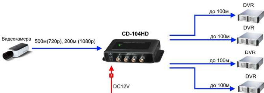
Рис. 3 Схема подключения приемника CD104HD
