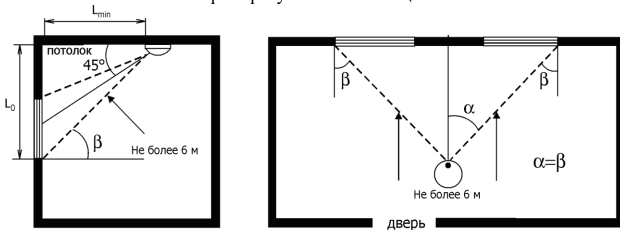
Рисунок А.1 – Установка на потолке
