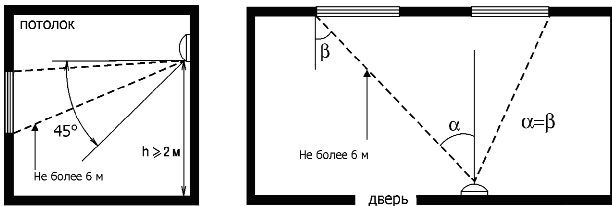
Рисунок А.2 – Установка на противоположной стене
